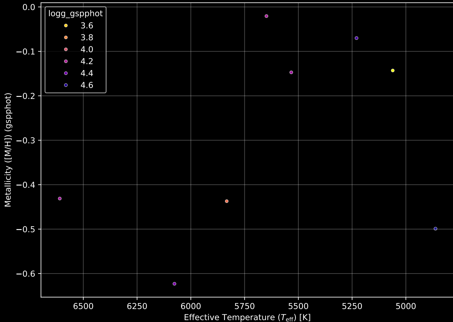
GALAH DR4 Field: [7368] Stellar Population Parameters (n= 8)
